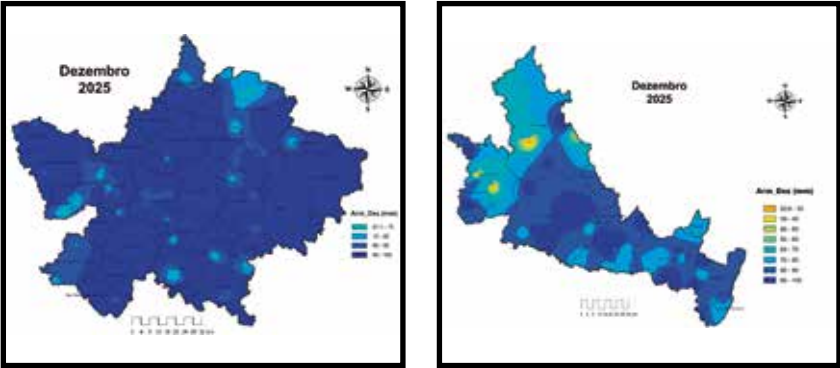
DISTRIBUIÇÃO DE ARMAZENAMENTO DE ÁGUA NO SOLO NA ÁREA MONITORADA DA COOXUPÉ SUL DE MINAS E CERRADO DO MÊS DE DEZEMBRO DE 2025
